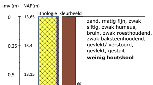
Boring 3 RD-coördinaten: 217841/441307
