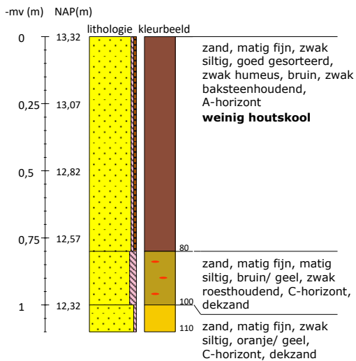
Boring 1 RD-coördinaten: 217791/441325
