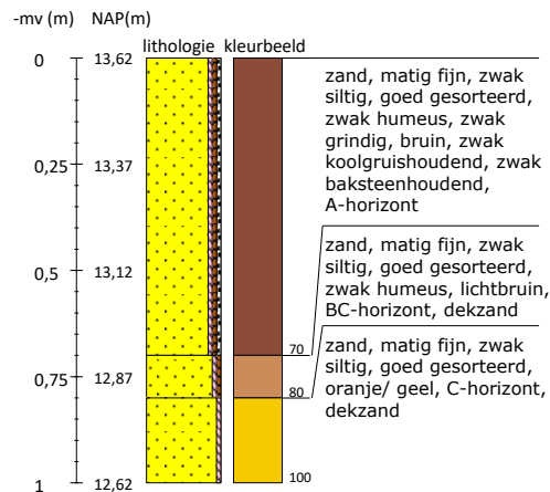
Boring 2 RD-coördinaten: 217812/441346
